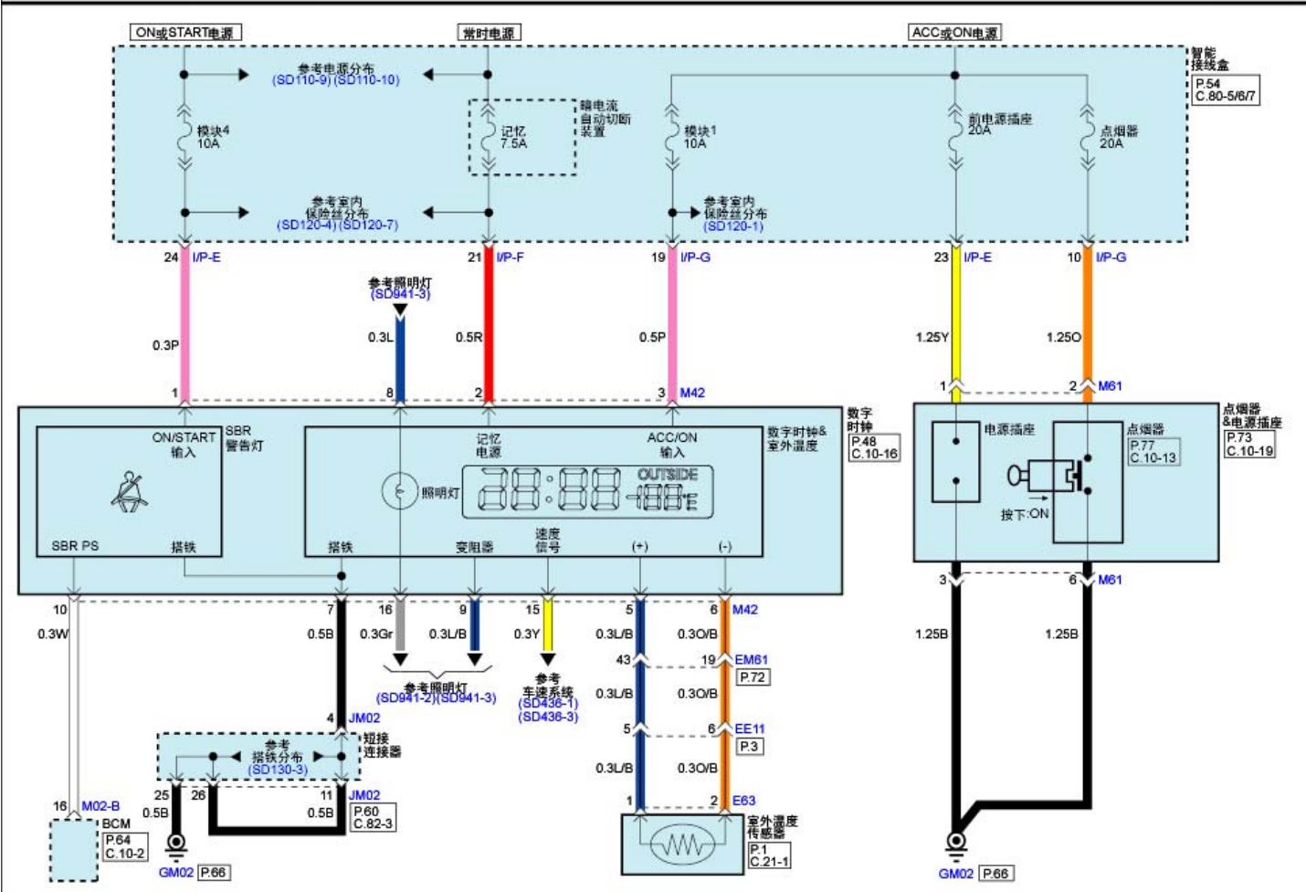
时钟&点烟器(电源插座)系统(1)
